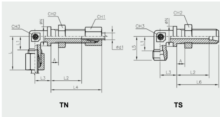
TN/TS 118 - Raccordo di attraversamento a gomito - Bulkhead Elbows
